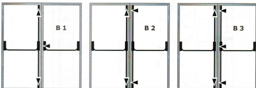
Wersja B - drzwi dwuskrzydłowe z przymykiem
